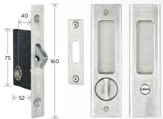
Sliding Door Privacy Set - Square Edge 70187 70188 70190
