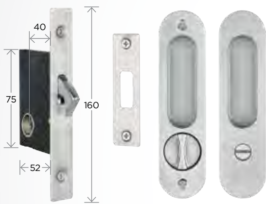
Sliding Door Privacy Set - Round Edge 70185
